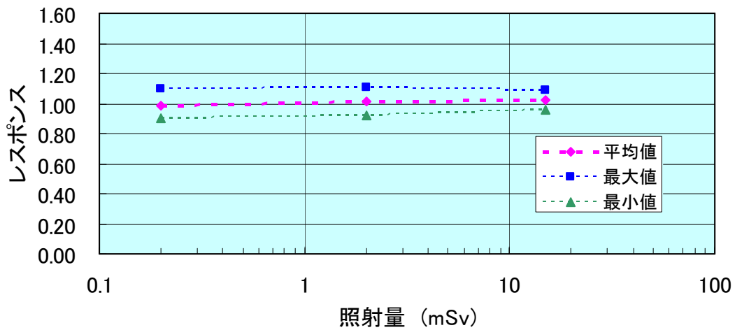
(1)線量直線性(34.9keV X線)
