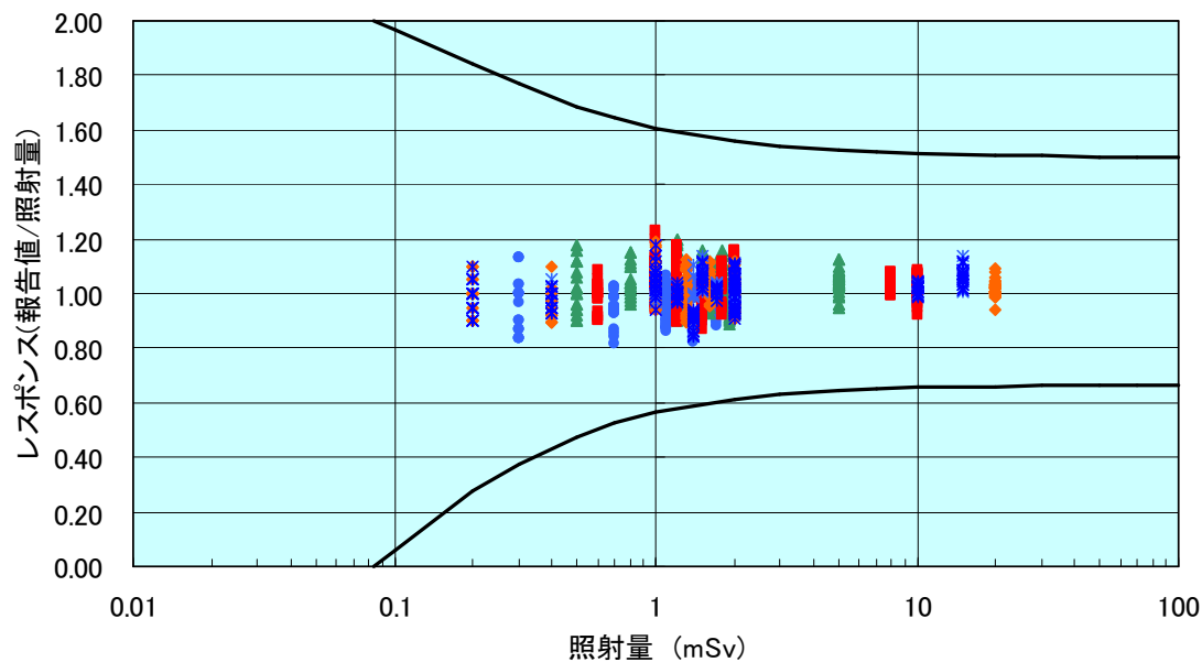
(1)X・ \gamma 線に対する測定精度
