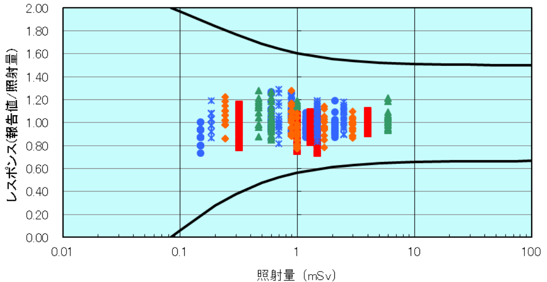
(2) 中性子に対する測定精度
