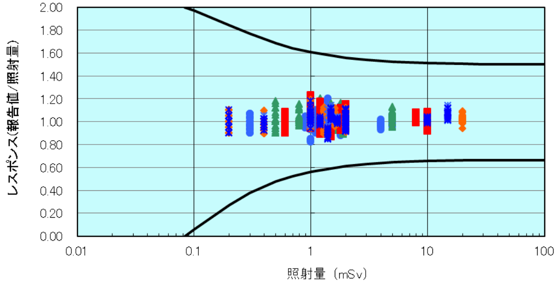
(1) X・γ線に対する測定精度
