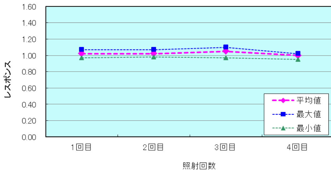
測定精度の安定性(Cs \gamma 線)
